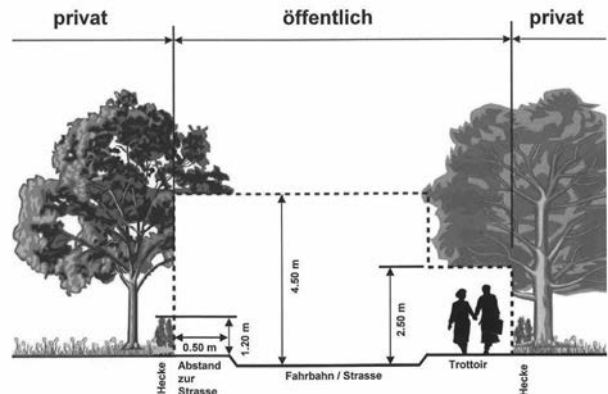
Lichtraumprofil bei Verkehrsflächen
