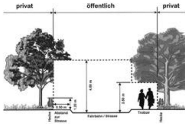
Lichttraumprofil bei Verkehrsflächen
