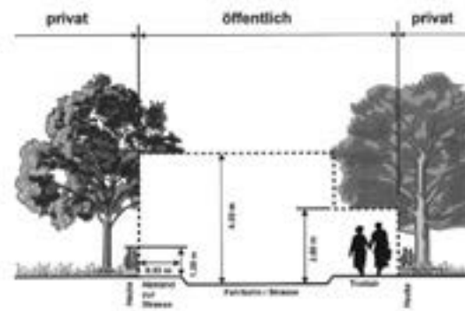
Lichtraumprofil bei Verkehrsflächen
