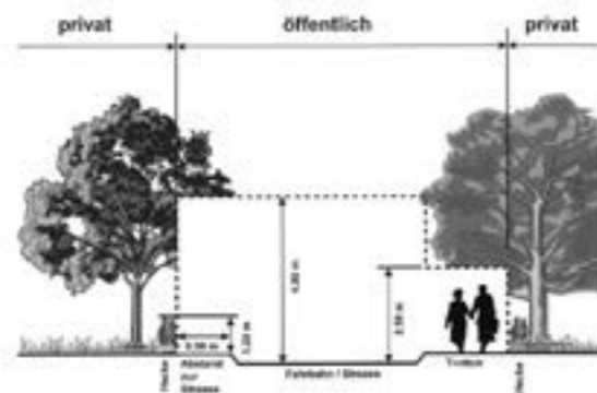
Lichtraumprofil bei Verkehrsflächen
