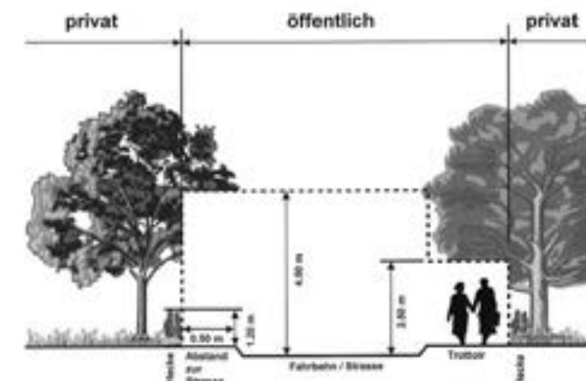
Lichttraumprofil bei Verkehrsflächen
